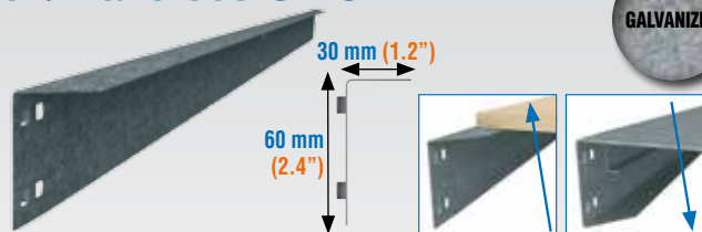
Larguero Serie L95 - Beam L95 Series
