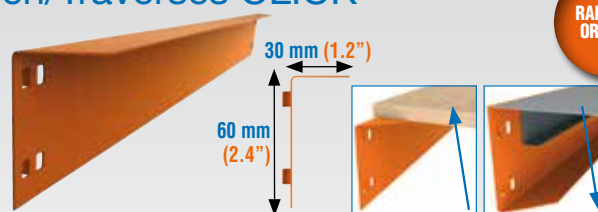
Largero Serie L95 - Beam L95 Series
